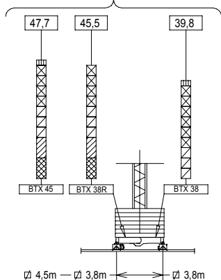
(H) TRASLACIÓN / TRAVELLING /
