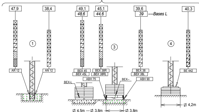
(H) ESTACIONARIA / STATIONARY /
